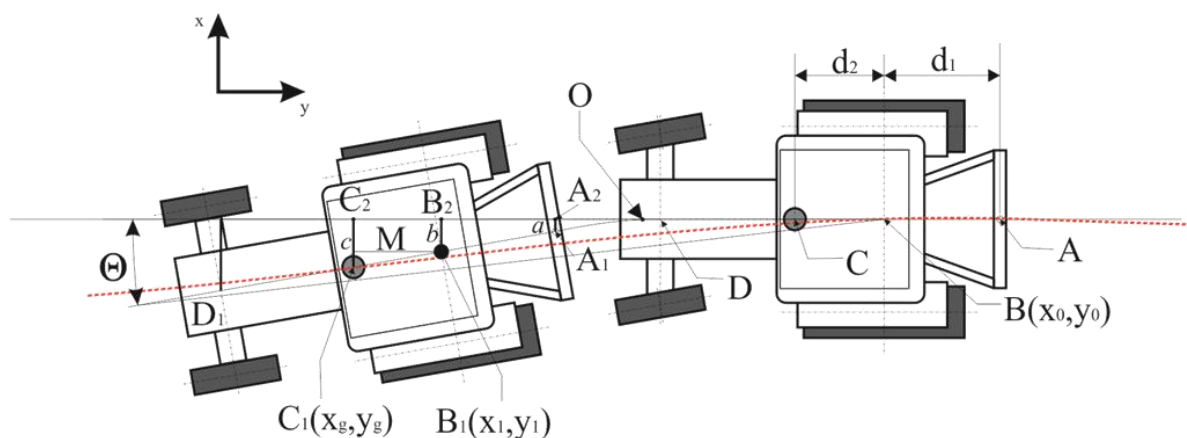
Slika 1.9. Šematski prikaz pomenosti traktora od idealne putanje vođenja ( Kostić et al., 2015a ) prijemnika i karakterističnih dimenzija traktora (slika 1.9).
