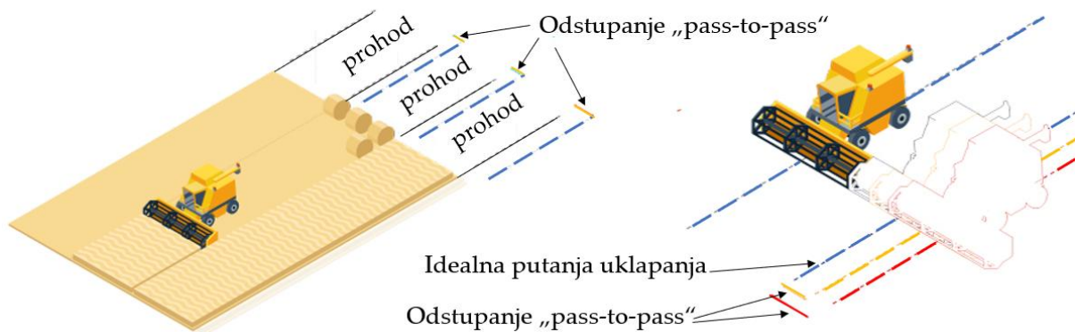
Slika 1.8. Greška nastala u navođenju mašina kao posledica pass-to-pass greške
